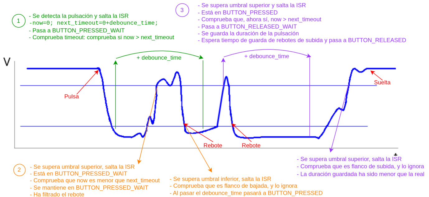
Ejemplo de 2 rebotes en una pulsación con tiempo de anti-rebotes bajo.
