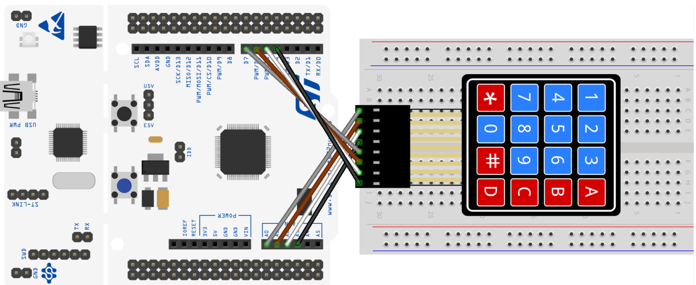
Montaje del teclado matricial con la Nucleo-STM32F446RE
