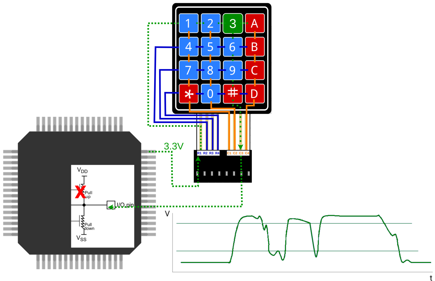
Ejemplo de excitación de fila R1, pulsando tecla 3, generando interrupción en pin conectado a columna C3.
