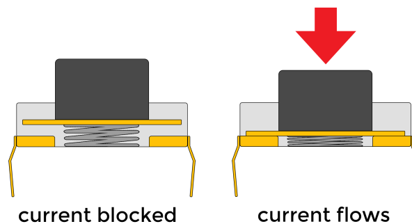
Representación mecánica de un botón.
