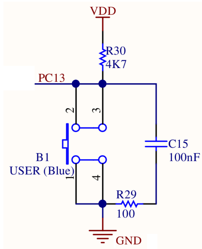
Esquema del circuito del botón en la placa Nucleo-STM32F446RE .
