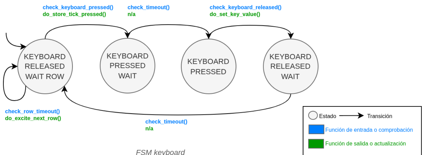
Máquina de estados del teclado matricial.
