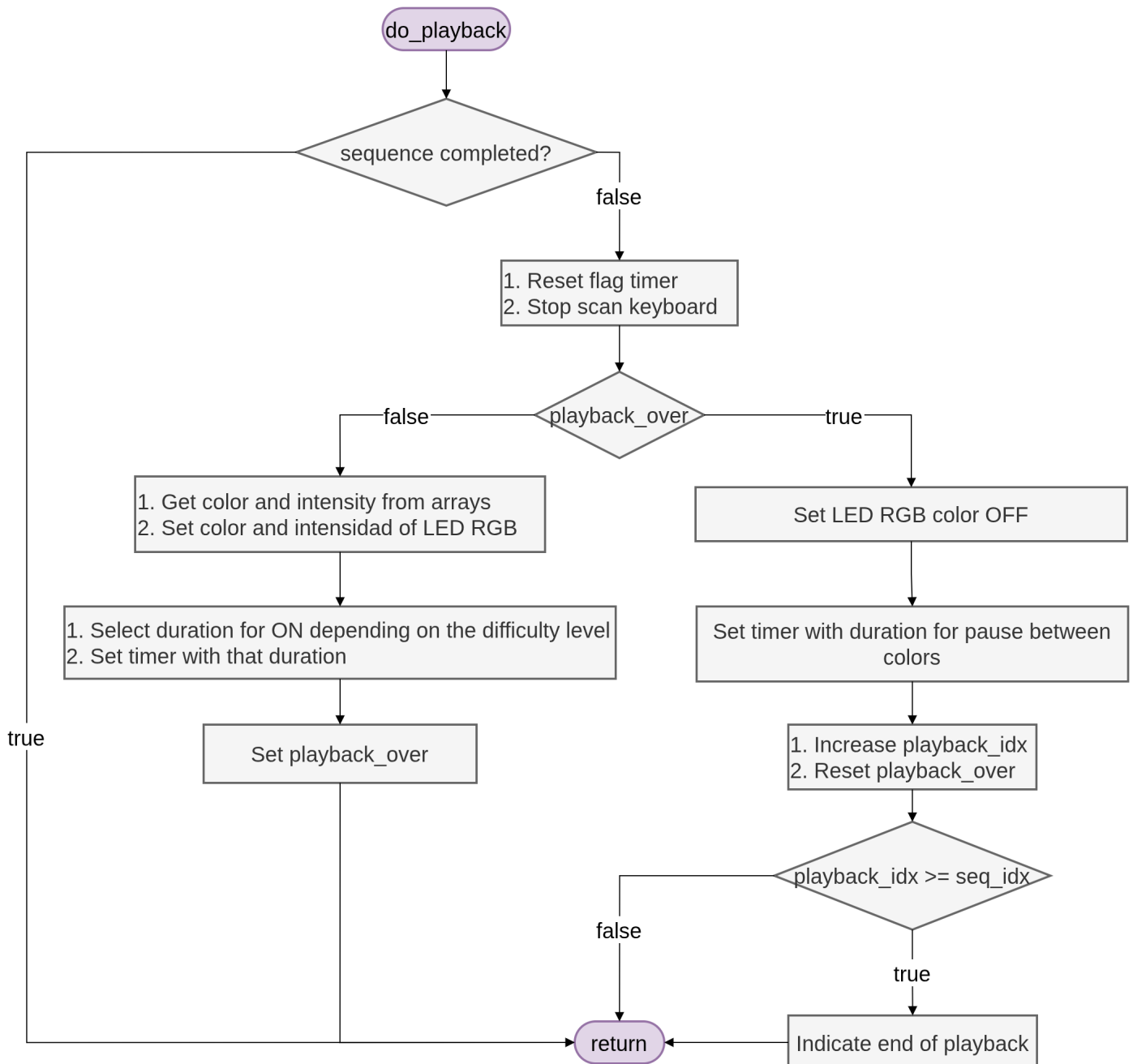
Diagrama de flujo de la función `do_playback()`.
