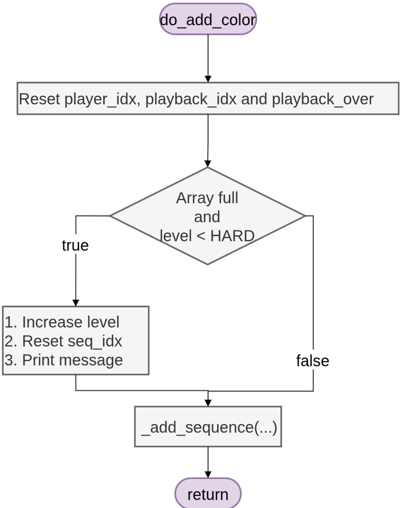
Diagrama de flujo de la función `do_add_color`.
