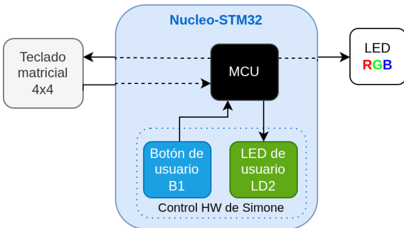
Diagrama de elementos del sistema.
