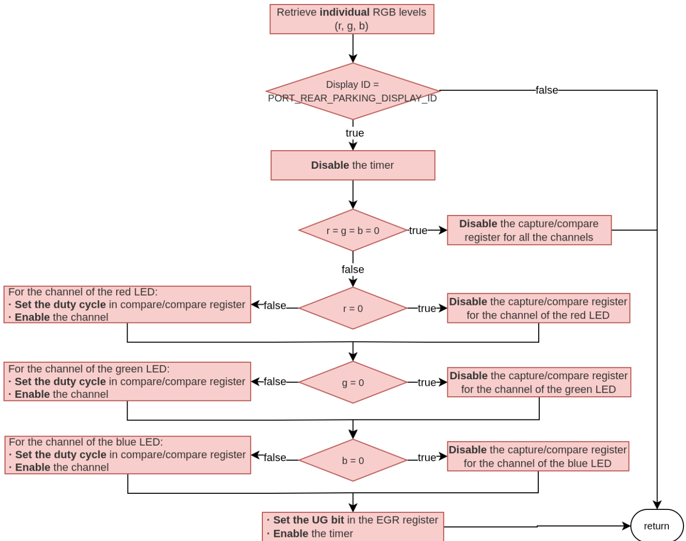
Flujograma de la función port_rgb_light_set_rgb() .
