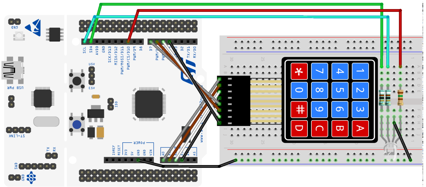
Montaje final con el teclado, el botón y el LED RGB.
