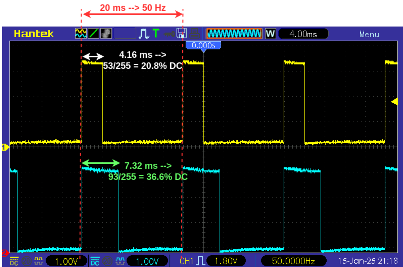
Ejemplo de señales PWM para un color amarillento.
