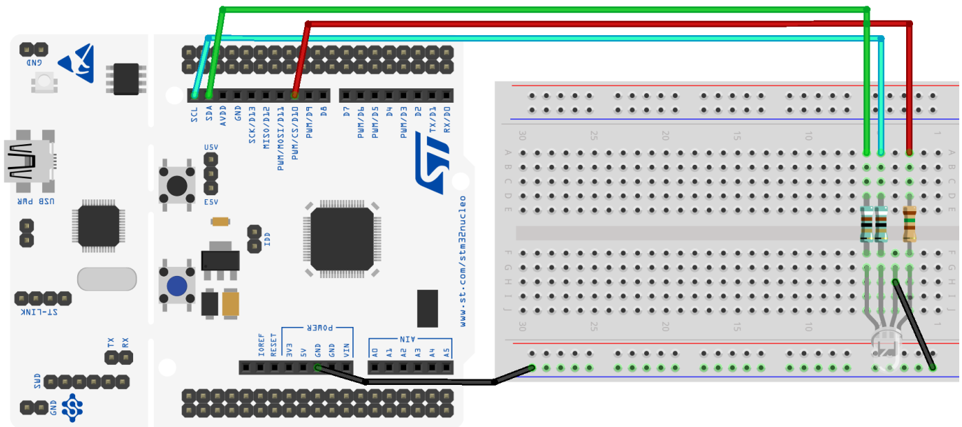
Montaje del LED RGB de cátodo común con la Nucleo-STM32F446RE.
