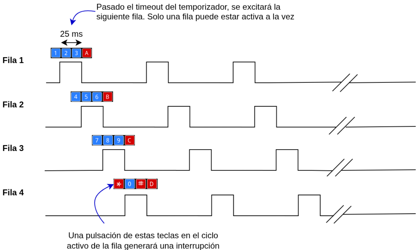
Diagrama de temporización de excitación de filas.
